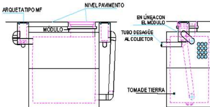
CONTENEDOR PARA DOS NODOS
